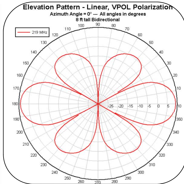
E-Plane / Elevation
