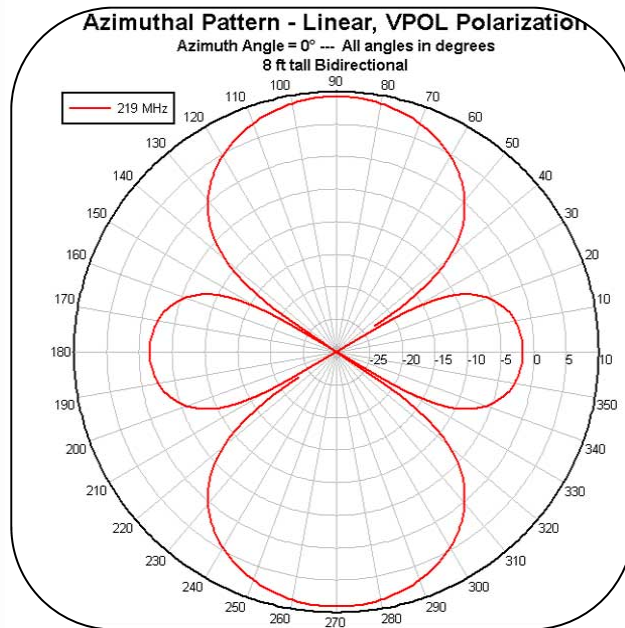
H-Plane / Azimuth
