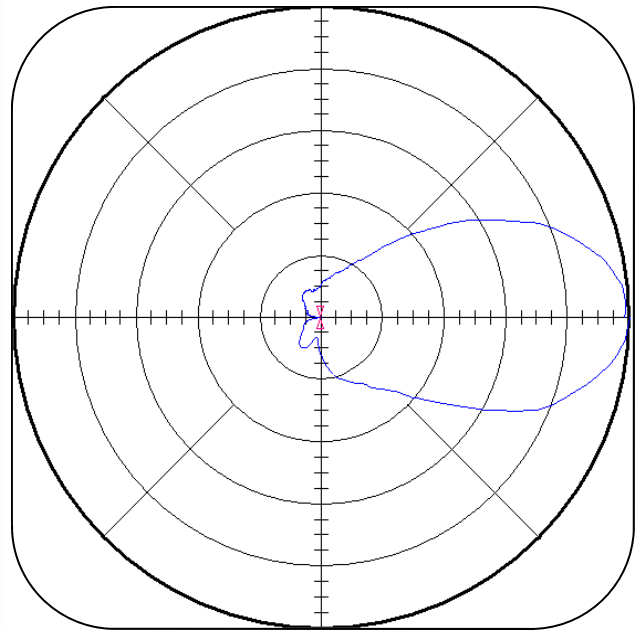
H-Plane / Azimuth
