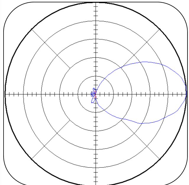
E-Plane / Elevation
